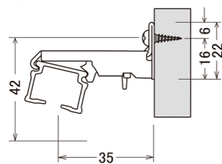
完全ワンタッチシングルブラケット
