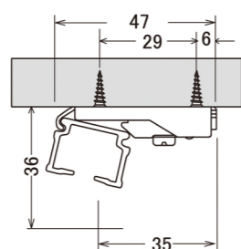
天井シングルブラケット
