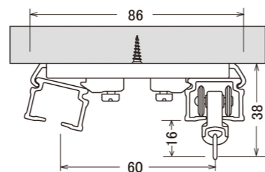
天井ダブルブラケット
