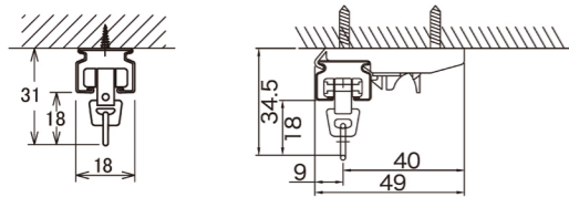
レール直付 天井付シングルブラケット
