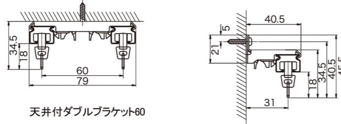
正面付ダブルブラケット60 正面シングルブラケット30
