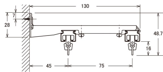
正面付ダブルブラケット75(公団用)
