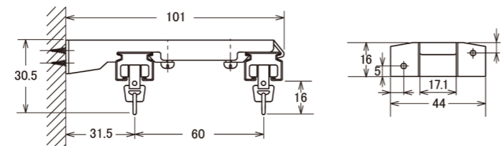
正面付ダブルブラケットT ブラケット幅: 44mm
